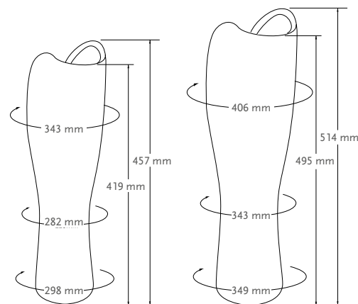
製品番号 2075R レギュラー
