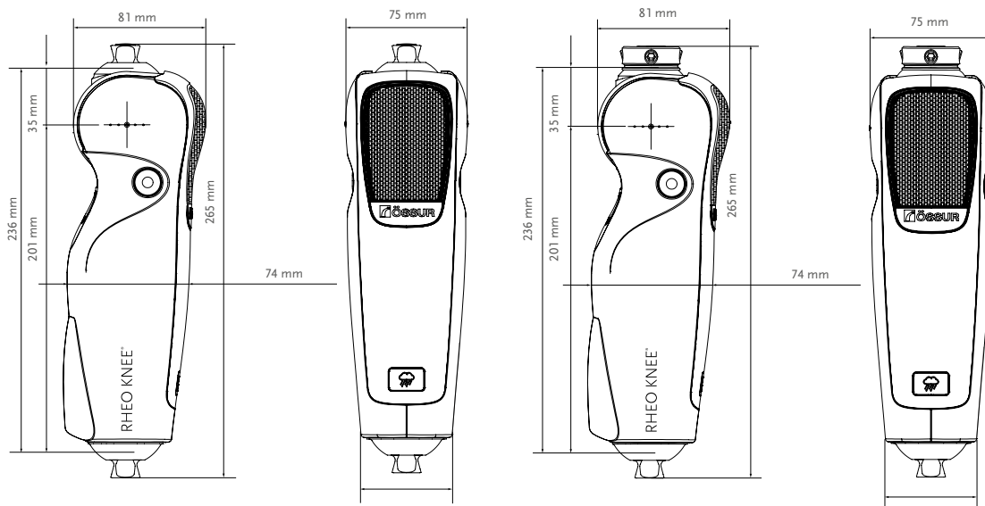
RHEO KNEEねじ切りトップアダプタ付(A - 145310)
